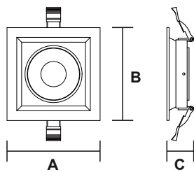
HV-BG102-FRAME-1-Anti
