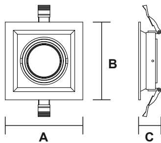
NR-BG102-FRAME-1
