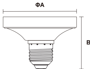
E27 TO GX53 Item Code:NR-E27-GX53
