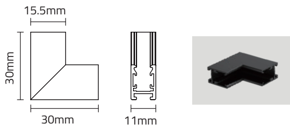
Model No:NR-ST-552TRA-L
