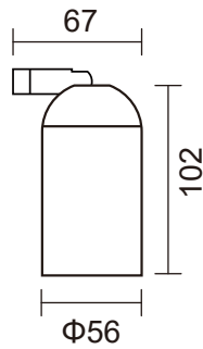
NR-TYD-MR16-A
