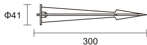
NR-TYD-REF
