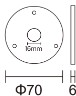
NR-TYD-REF-16mm
