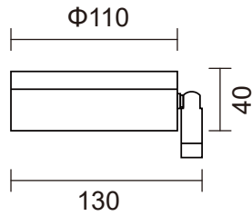
NR-TYD-GX53-100-A
